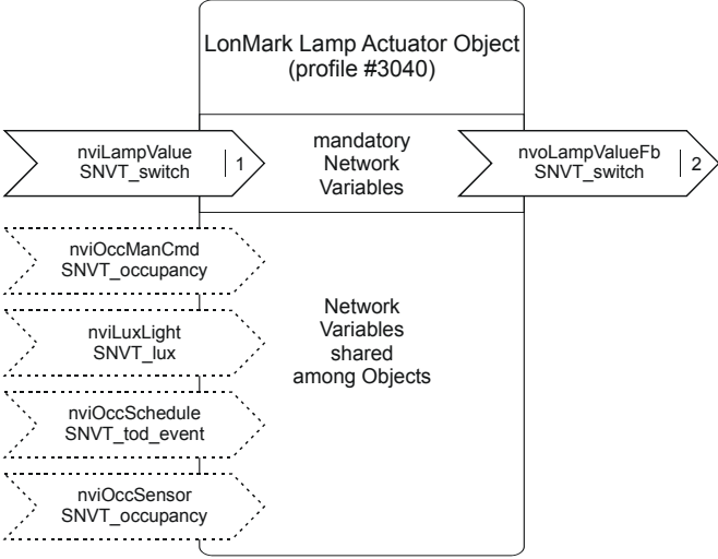
Fig. 12. Lamp Actuator Object
