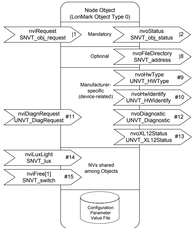
Fig. 10. Node Object
