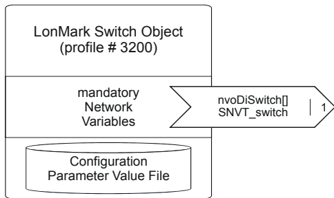
Fig. 7. Switch Object
