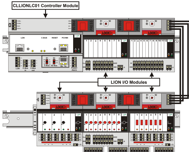
Fig. 8. LION Controller and I/O Modules on DIN rails
