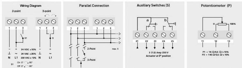
Standard, 2- és 3-pont működésű villamos zsalumozgatók
