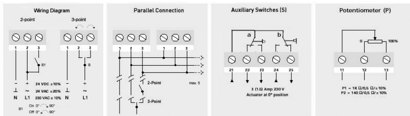
Villamos bekötés
